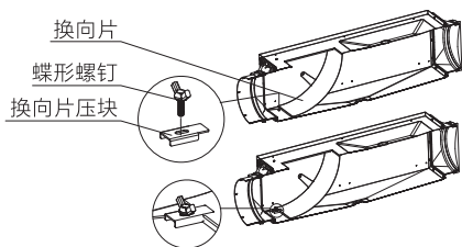
图（3）左侧出风换向片安装示意图
