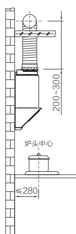
图 (2) 橱柜安装 侧视图
