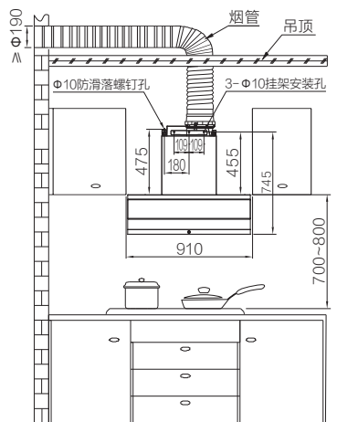
图 (1a) 橱柜挂架安装 正视图 (标配)
