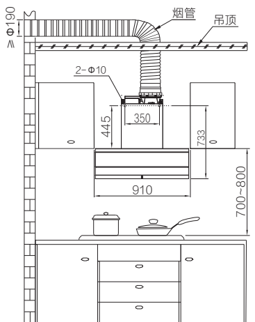
图 (1b) 橱柜平推安装 正视图 (选配)
